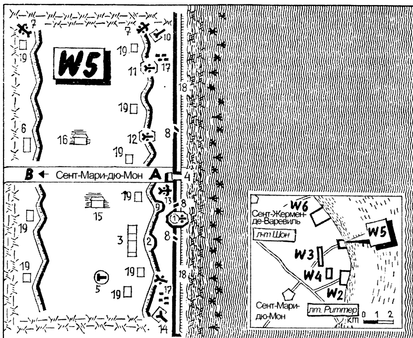
План оборонительной позиции W 5 на побережье у Эббе
