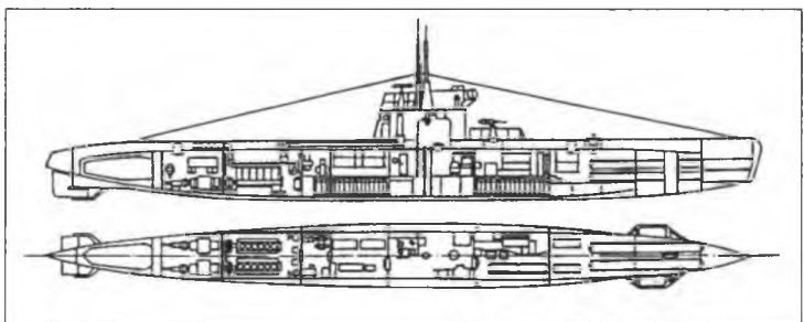
Подводная лодка М-200 в разрезе
