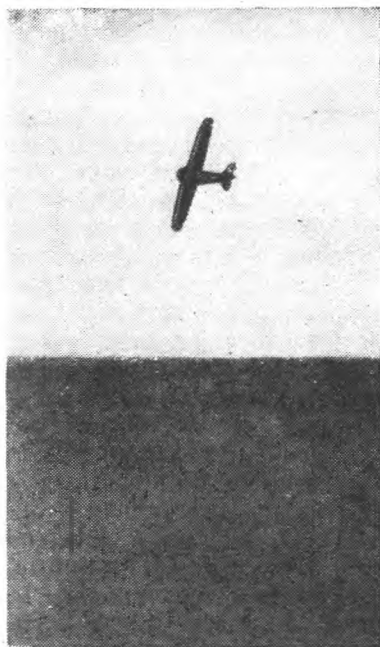
Самолет П. Н. Нестерова над Курневским аэродромом в Киеве и схема мертвой петли, впервые выполненной им в 1913 г. (воспроизведение собственноручного чертежа П. Н. Нестерова)
