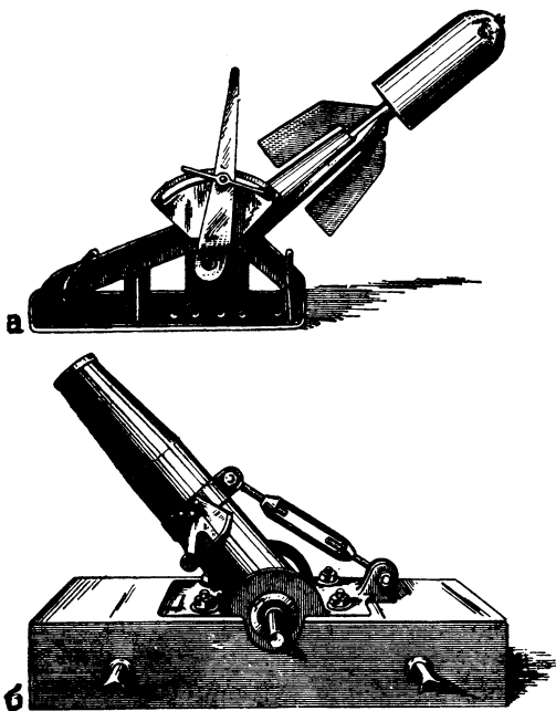
Минометы: а — 47-мм миномет системы Лухонина; б — 58-мм миномет типа Ф. Р.
